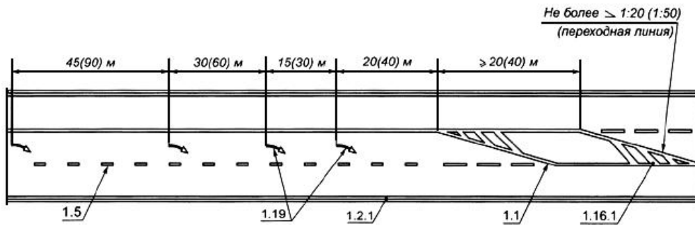
Рисунок В.8 - Пример нанесения разметки при уменьшении количества полос для движения в одном направлении
